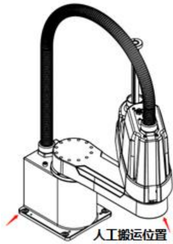
图 1.1 GBT-S6A 转运姿态
