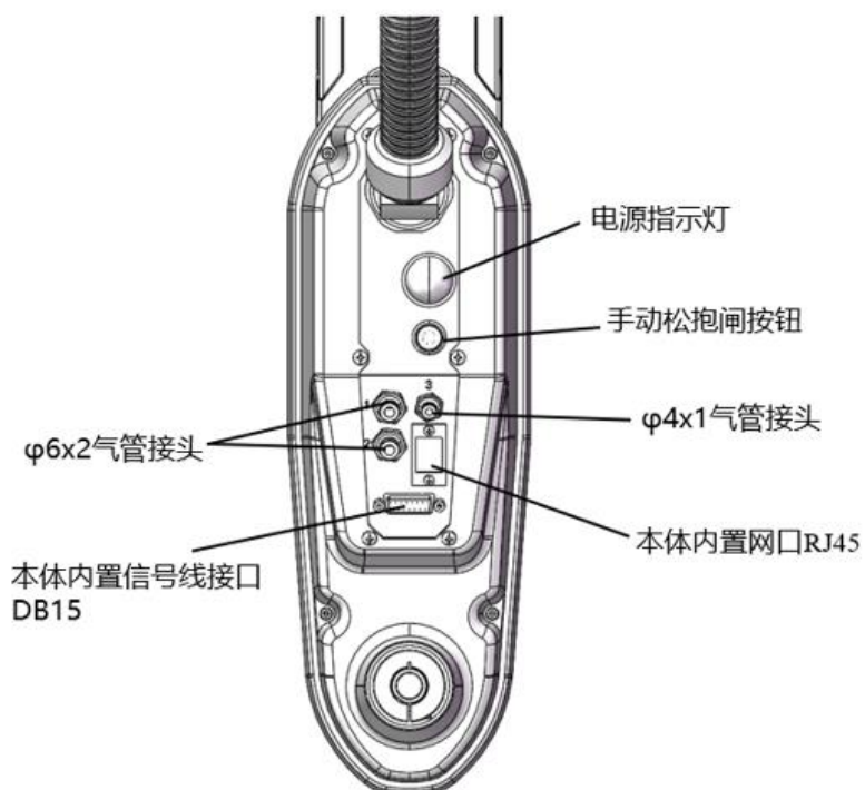
图 5.2 手臂气管和电气接口位置
