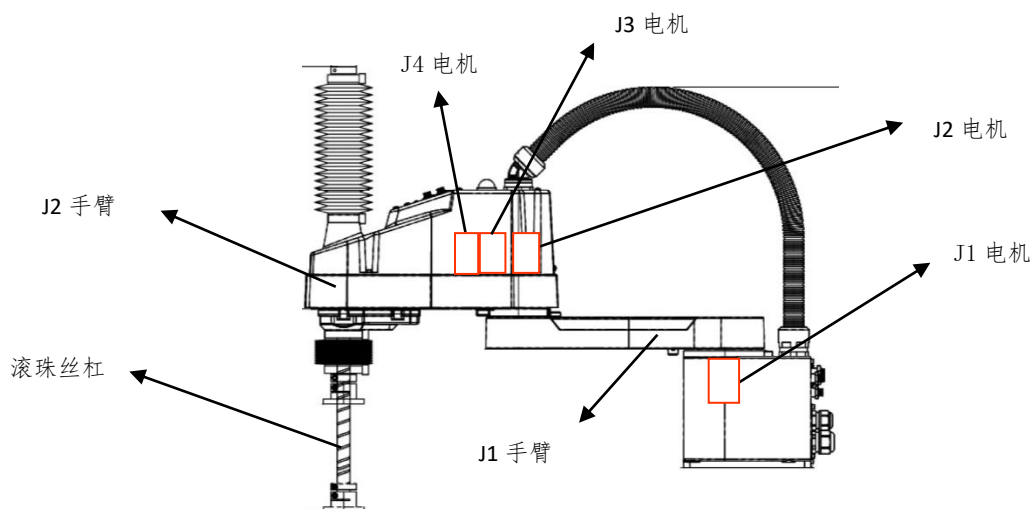
图 3.1 GBT-S6A 机器人电机位置示意图
