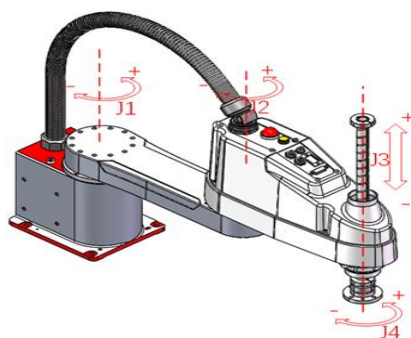
图 3.2 GBT-S6A 各运动关节及运动正方向
