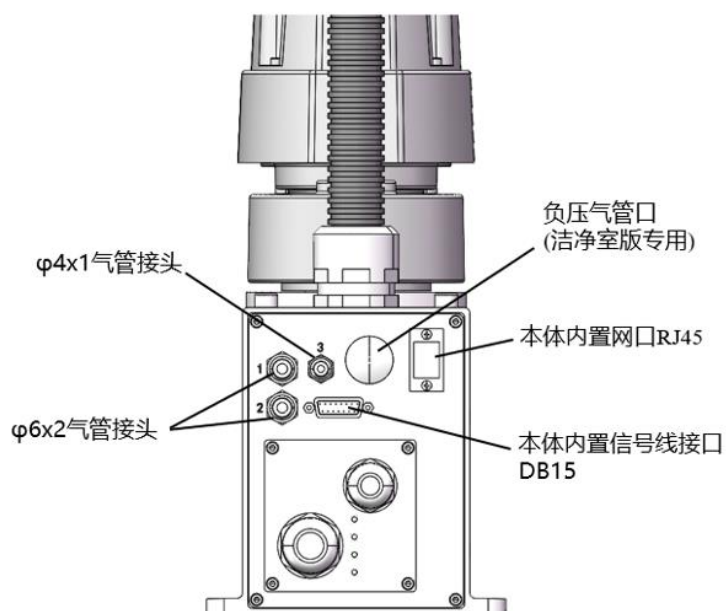
图 5.1 底座气管和电气接口位置
