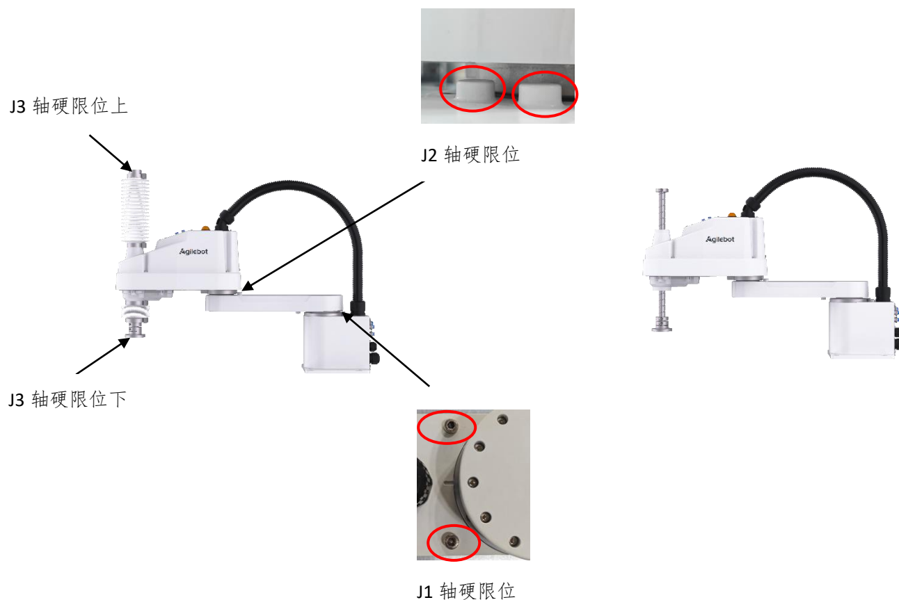
图 3.6 GBT-S6A 系列硬限位图（左图为洁净版，右图为标准版；硬限位相同）
