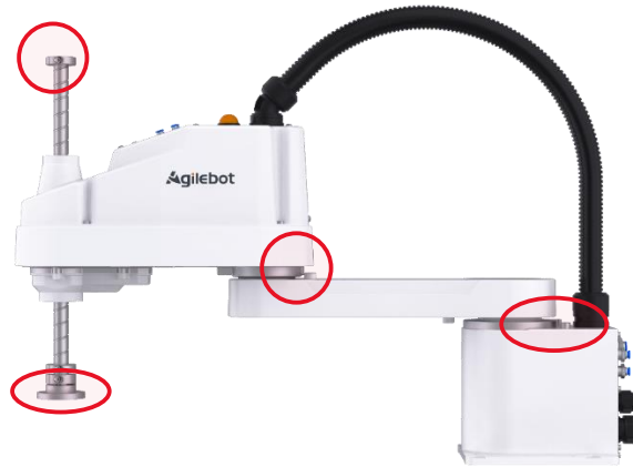
图 6.1 GBT-S6A 系列硬限位图
