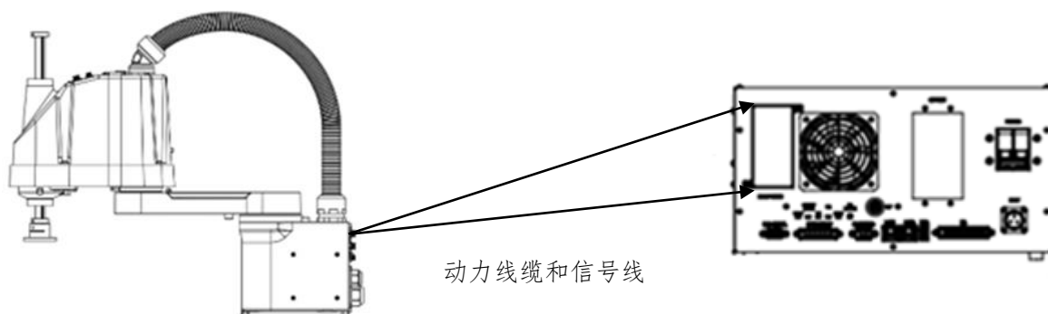
图 2.1 GBT-S6A 机器人与控制柜连接示意图
