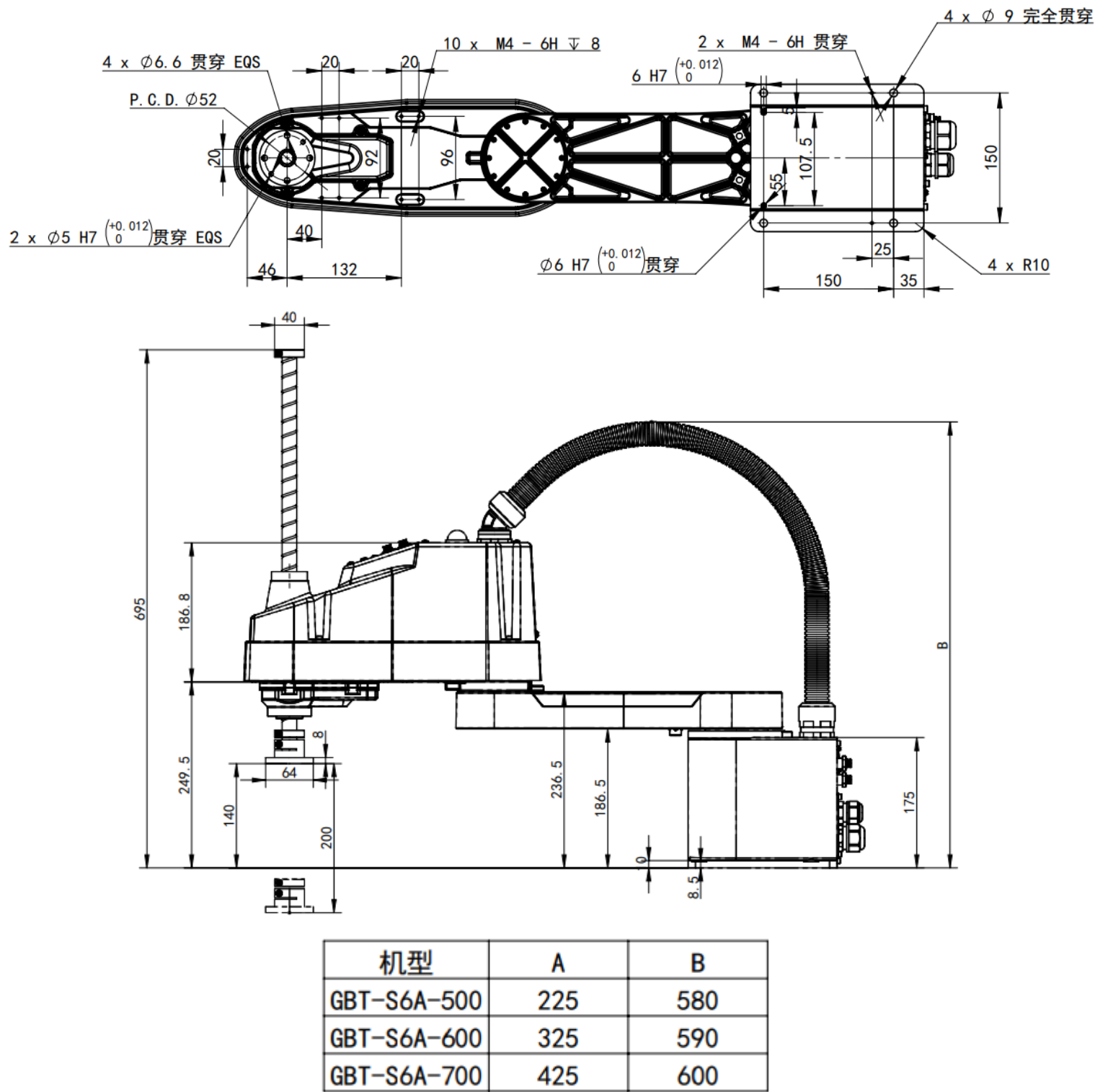
图 3.4 GBT-S6A 系列外形尺寸图
